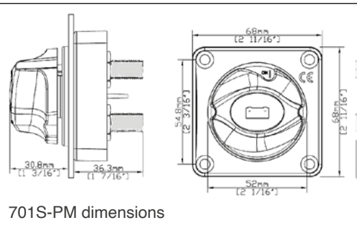
701-S dimensions
