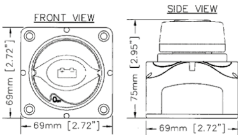
701 dimensions
