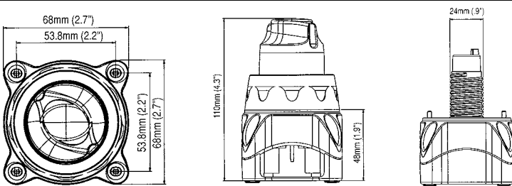
700 EASYFIT dimensions
