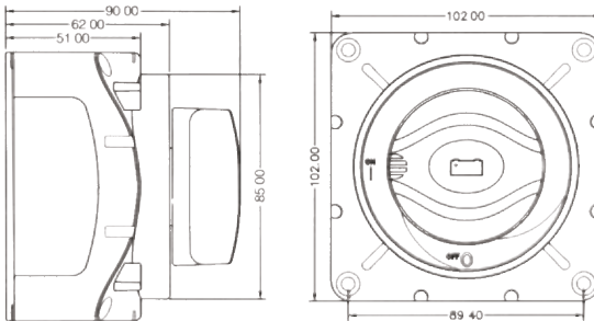
720 dimensions
