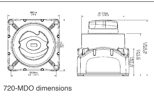
720-MDO
