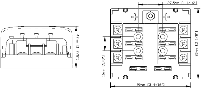
ATC-6W dimensions
