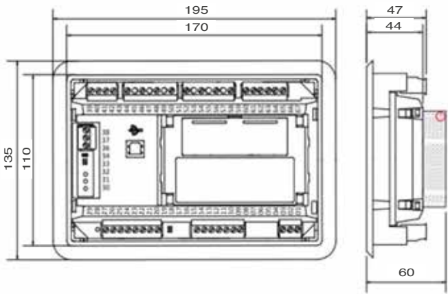
EOB-1500® Dimensions
