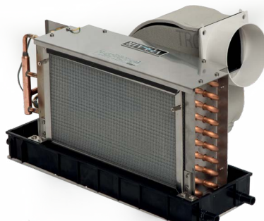
FANCOIL V12 - 12.000 BTU/h
