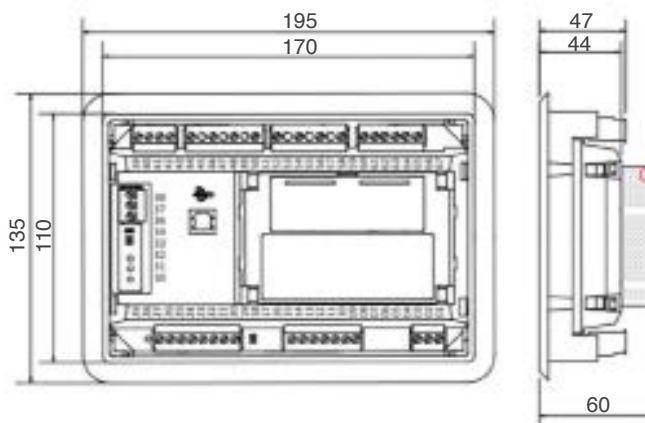
EOB-1500® dimensions
