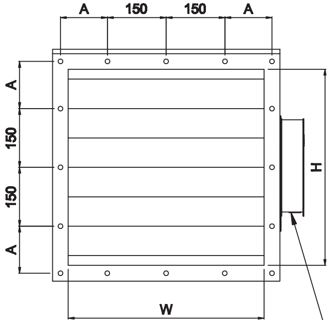
Attuatore elettrico / Electric actuator (24V-120V-230V)
